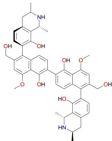
Jozipeltine A (32)
