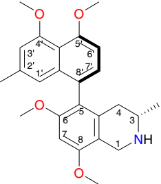
Ancistrobrevine (20)
