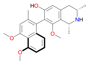
Ancistrobertsonine D (24)
