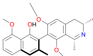
Ancistrocladinine (28)
