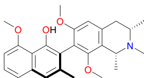
Ancistrotectorine (29)
