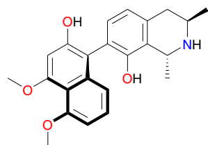
Habropetaline A (30)
