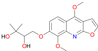
Evoxine (41)
