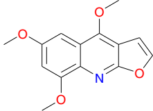
Maculosidine (38)
