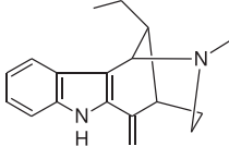
uleine (2)
