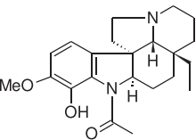
aspidoscarpine (1)
