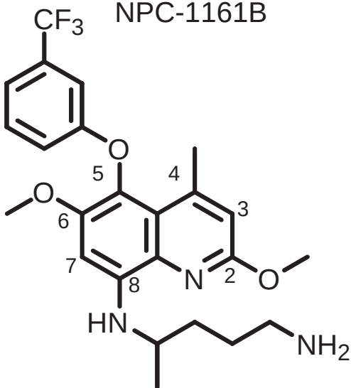
Tafenoquine
