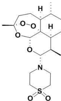
Artemisone
