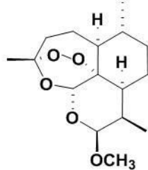
Artemether
