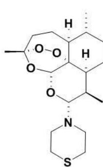
Artemiside
