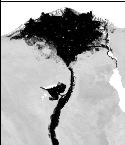
NDVI
