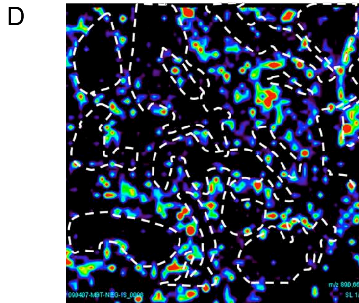
ST (d18:1/C24:0) m/z 890.6
