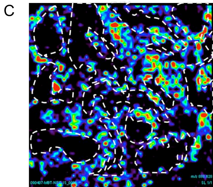
ST (d18:1/C24:1) m/z 888.6
