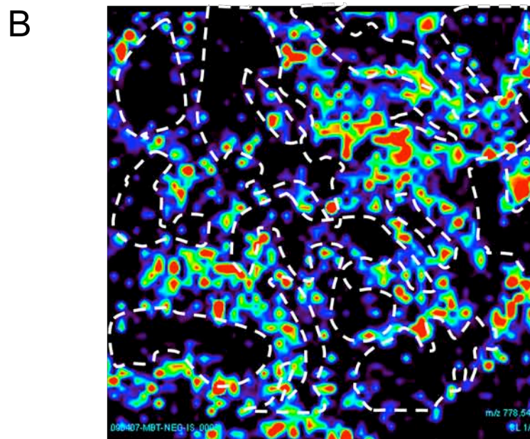
ST (d18:1/C16:0) m/z 778.6
