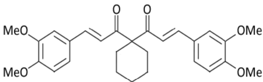
FLLL32
