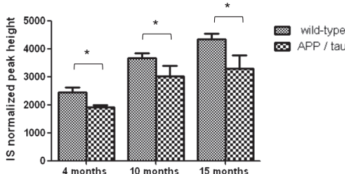
(B) 38:2pPE (p18:1/20:1)
