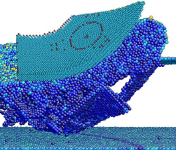
(a) Cu
