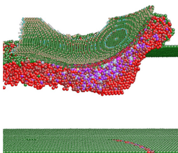
(b) Si
