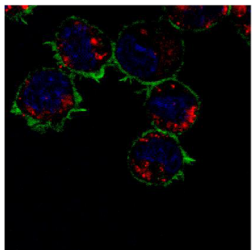
QD-PEG-COOH
