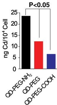
QD-PEG-NH 2
