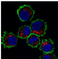
QD-PEG
