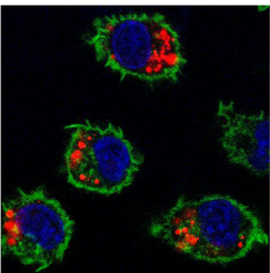
QD-PEG-NH 2
