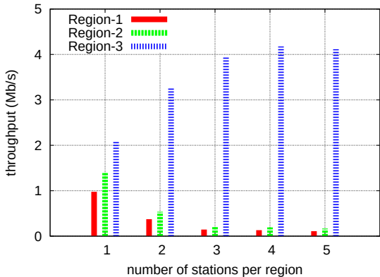
(a) IEEE 802.11
