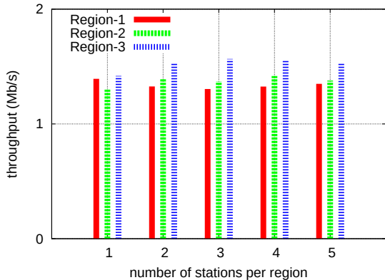
(b) TaLE
