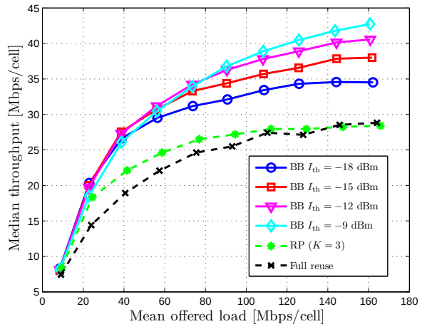
(d) Median cell throughput
