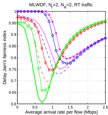
(d) Delay Jain's fairness index
