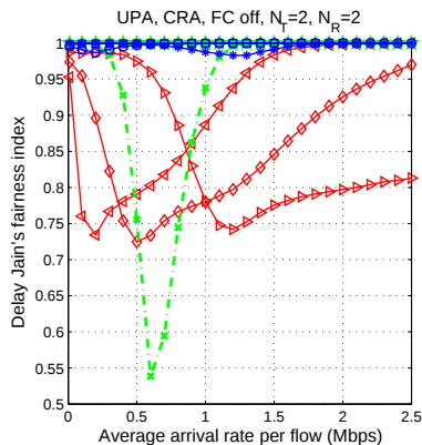
(d) Delay Jain's fairness index
