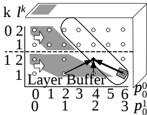
(d) 3D layer graph
