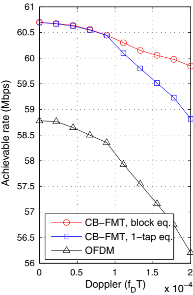
SNR=15 dB
