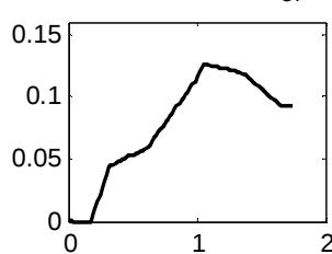
Glycogen r_{183}
