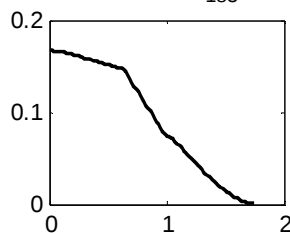
Glycogen r_{183}
