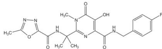
Raltegravir (MK-0518)
