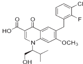
Elvitegravir (JTK-303)
