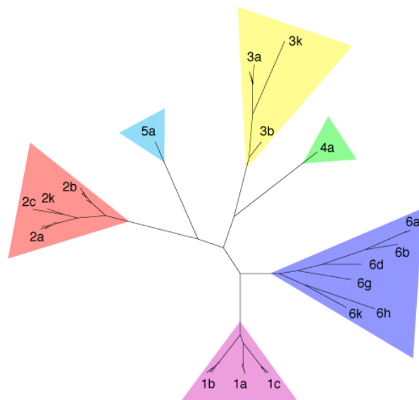
(d) Okamoto region of NS5B
