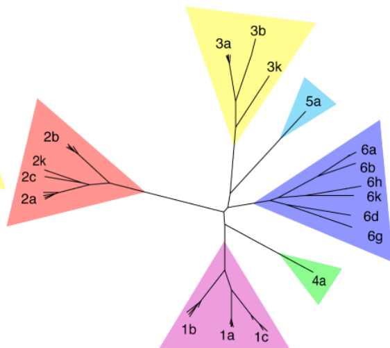
(d) Okamoto region of NS5B
