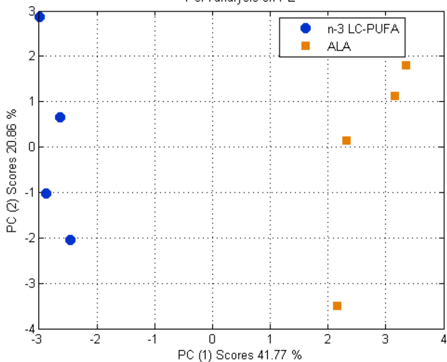
PCA analysis on PE
