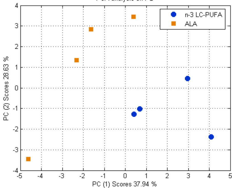
PCA analysis on PS
