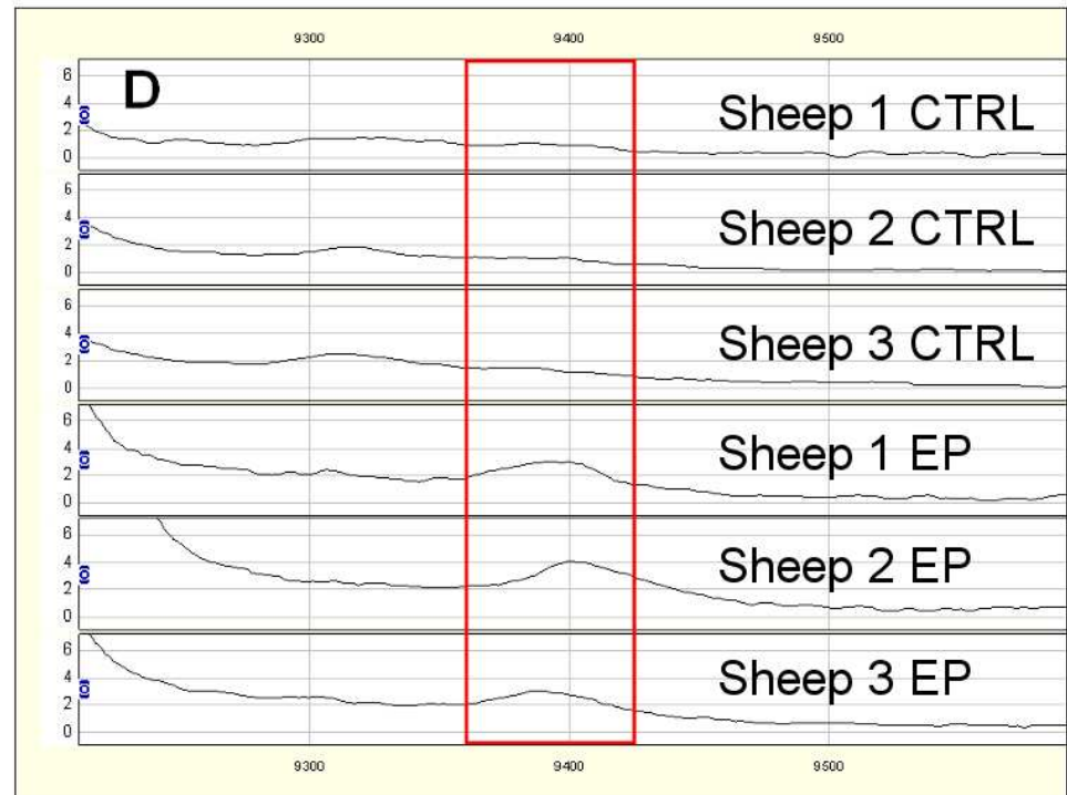
S4 9395 Da
