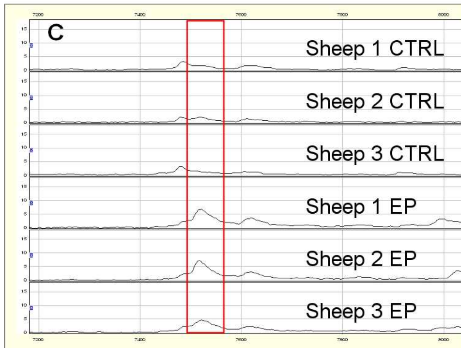
S3 7475 Da
