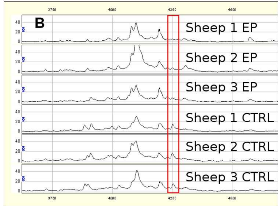
S2 4250 Da
