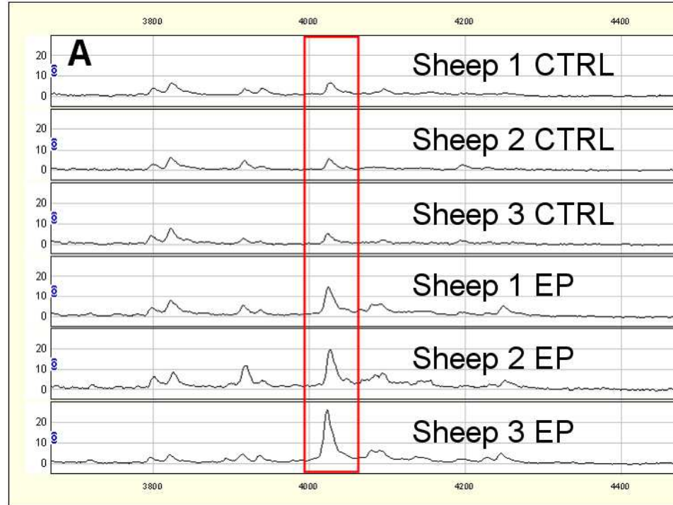
S1 4030 Da
