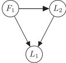
(ii) Adding an edge (F_1, L_2) .
