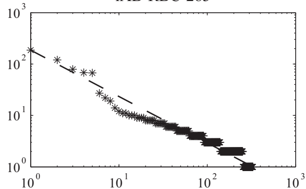
iAB-RBC-283
