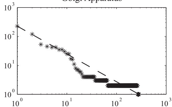
Golgi Apparatus
