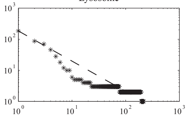
Lysosome
