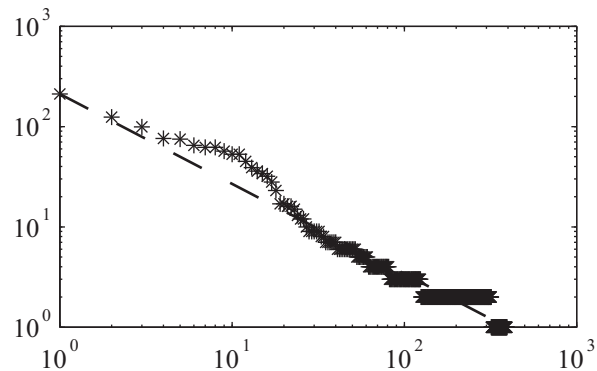
Mitochondria
