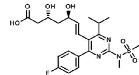
Rosuvastatin
