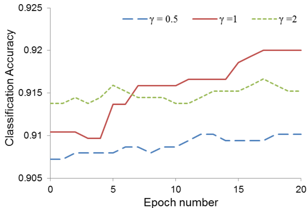
(b) Parameter learning
