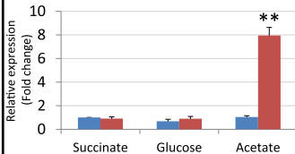
RSP_1939
