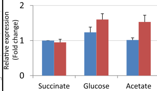
RSP_1146
