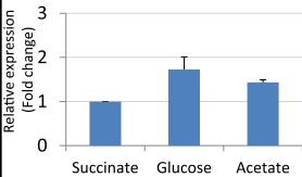
RSP_0240 (pntA)
