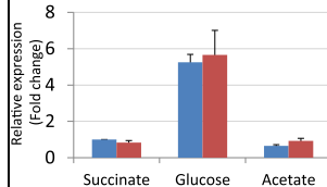
RSP_1146
