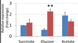
RSP_0661
