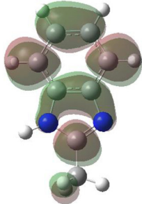
LUMO
