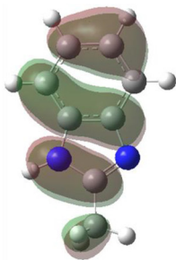
HOMO
