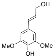
sinapyl alcohol, SA
