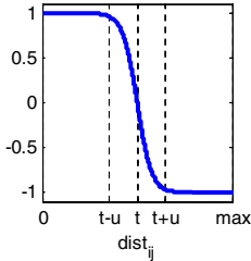
SWRF*
