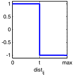
SURF*
