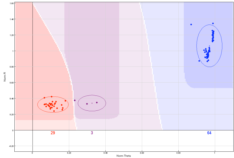
A. rs8081356
