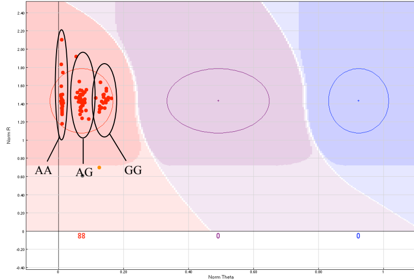
B. rs1632947
