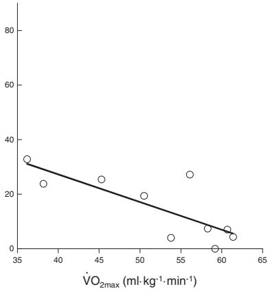
(b) HIAT
