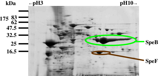
A (GT01 wild)
