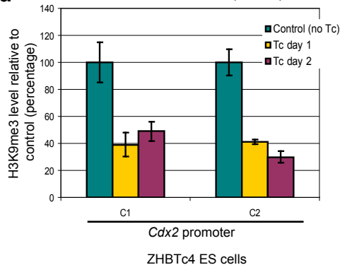
H3K9me3 carrier ChIP (Q-PCR)
