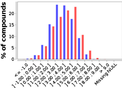
logP(o/w)
