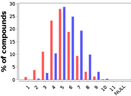
HBA
