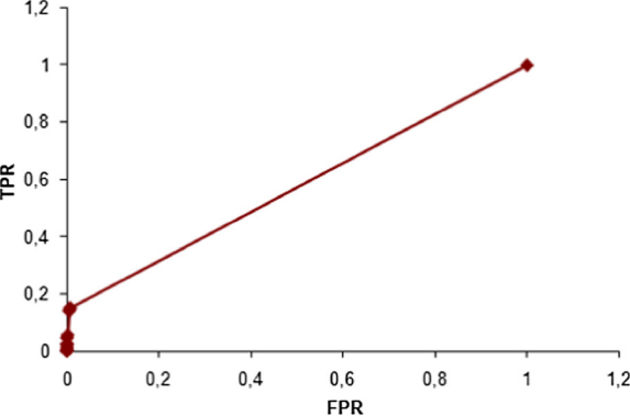
(a) ROCLLSVMW3xW2
