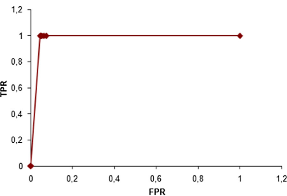
(b) ROCLLBayesW3xW2
