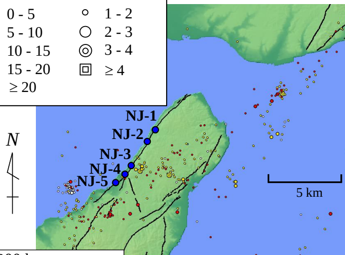
Nojima Fault (NJ)
