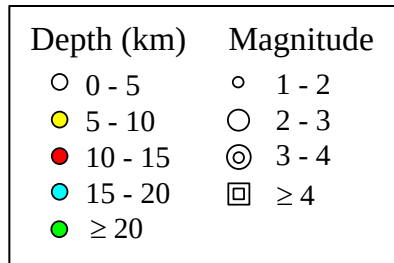
Nojima Fault (NJ)
