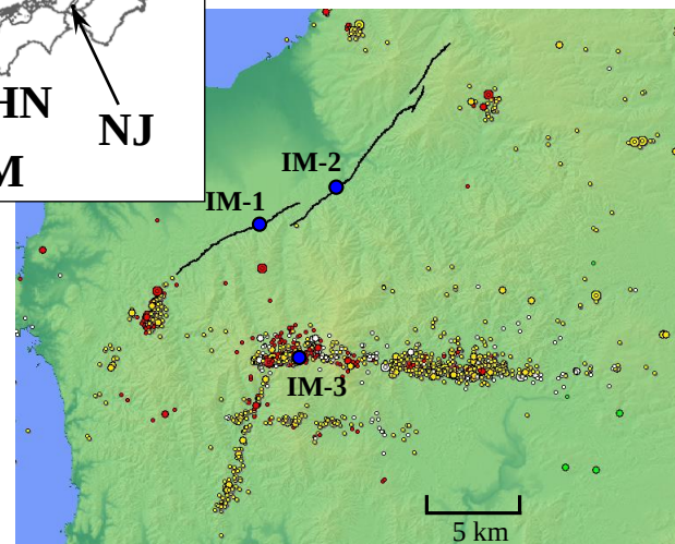
Izumi Fault (IM)
