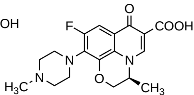
4 , Levofloxacin
