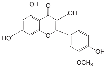
Isorhamnetin (3)
