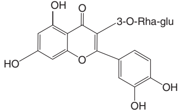
Rutin (2)
