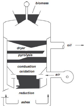
UPDRAFT
