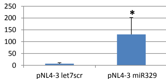
miR329
