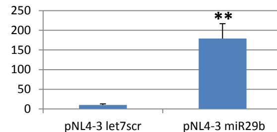
miR29b
