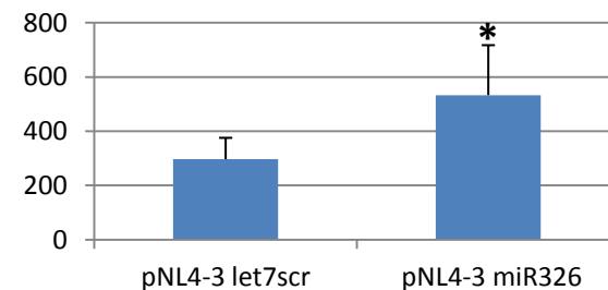
miR326
