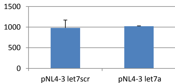
let7a
