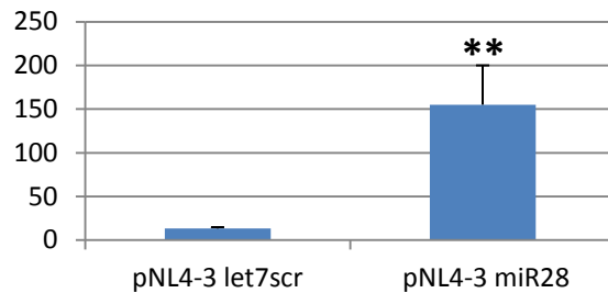
miR28
