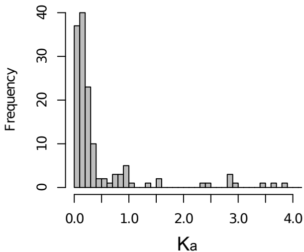
L. polyphemus paralogs - T. tridentatus orthologs
