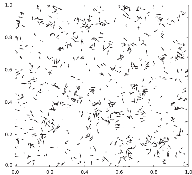
(d) High driving noise. \eta = 1.96
