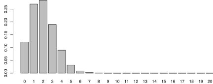
(a) Binomial distribution
