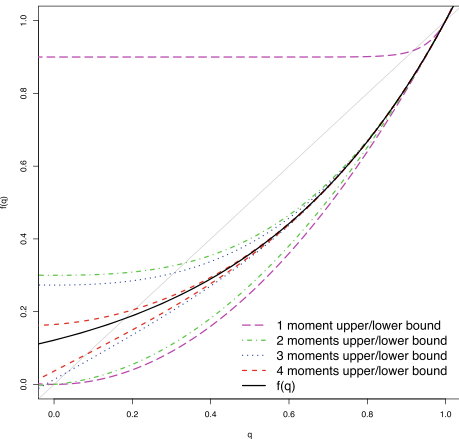
(a) Binomial distribution
