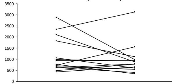
PCNA (201202)
