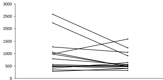
TYMS (202589)
