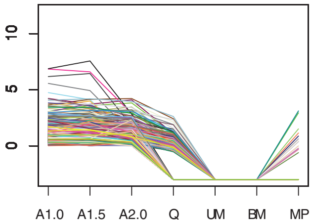
(d) Microspore maturation N=140
