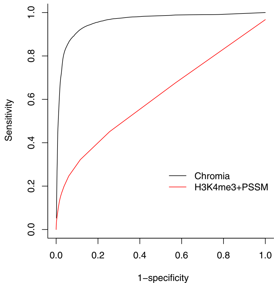
E2f1 promoter
