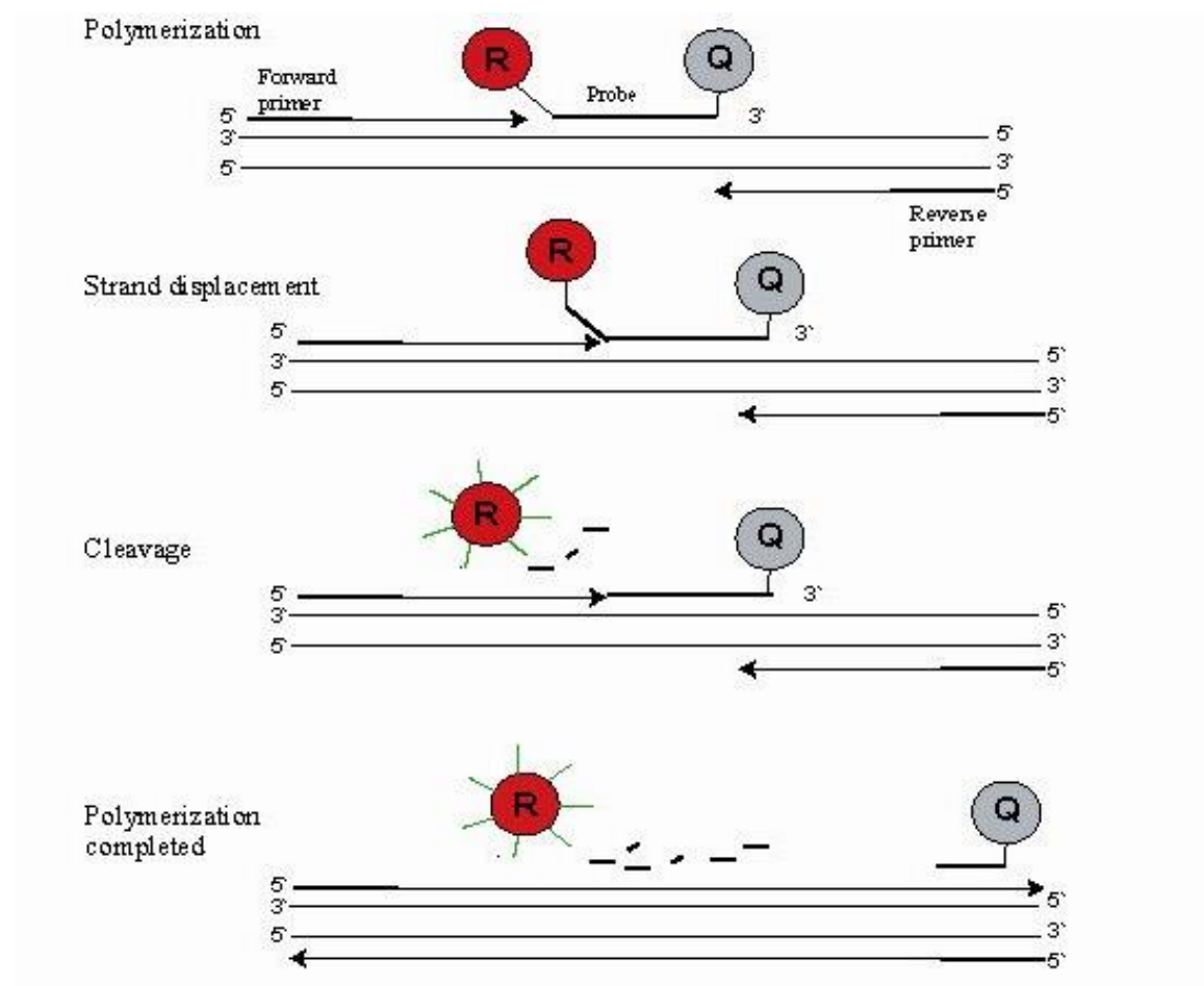
Fig.1.TaqMan assay.
