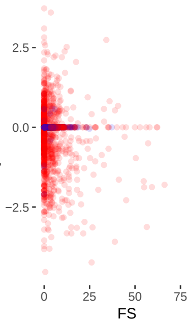
MQRankSum
