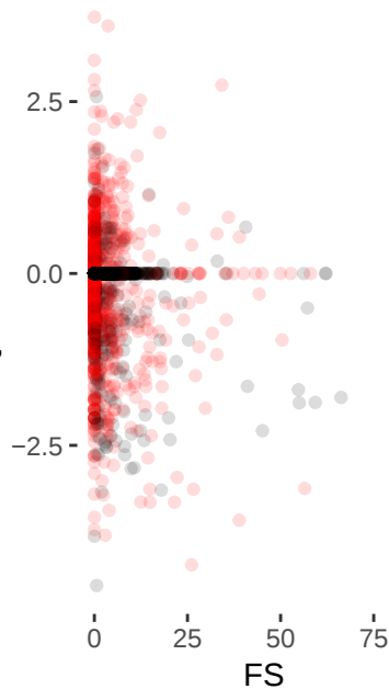
MQRankSum
