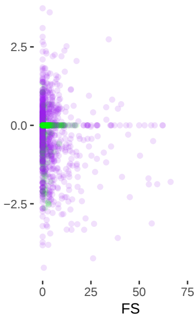
MQRankSum
